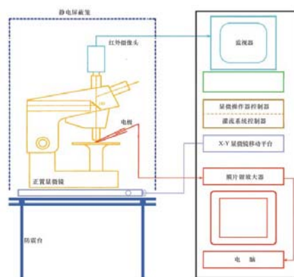
(脑片/组织切片膜片钳实验系统)
